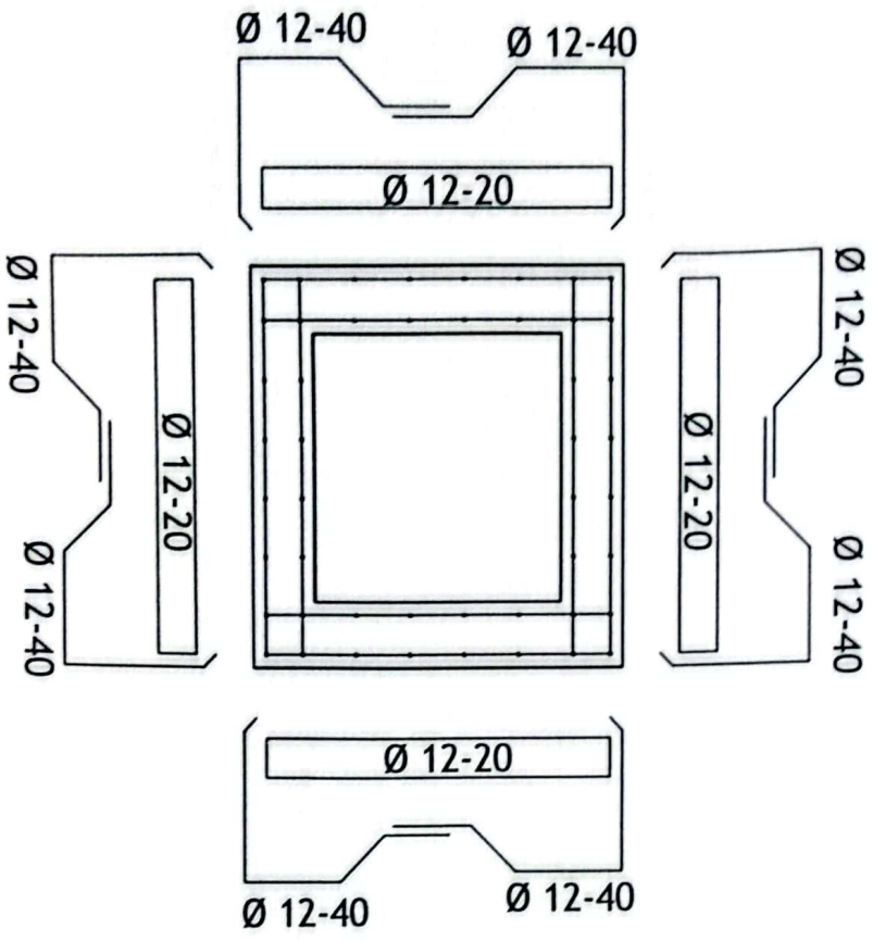
DETAIL PEMBERSIHAN BOX SKALA 1 : 30
