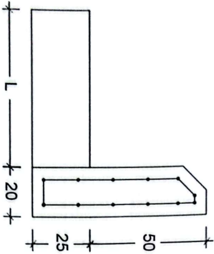
DETAIL - 01 SKALA 1:15
